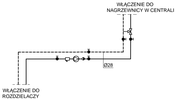
SCHEMAT PODŁĄCZENIA NAGRZEWNICY
