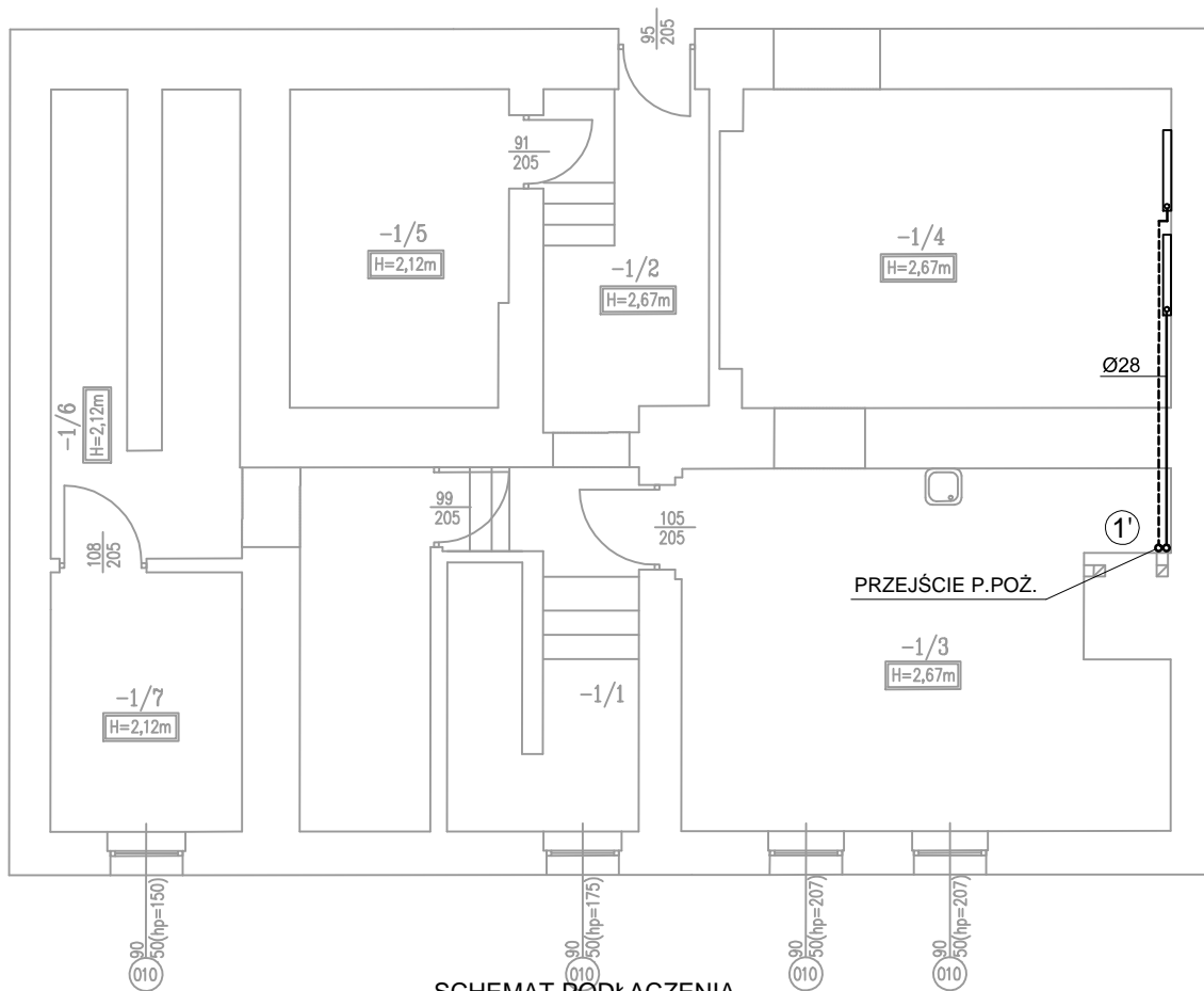
SCHEMAT PODŁĄCZENIA NAGRZEWNICY
